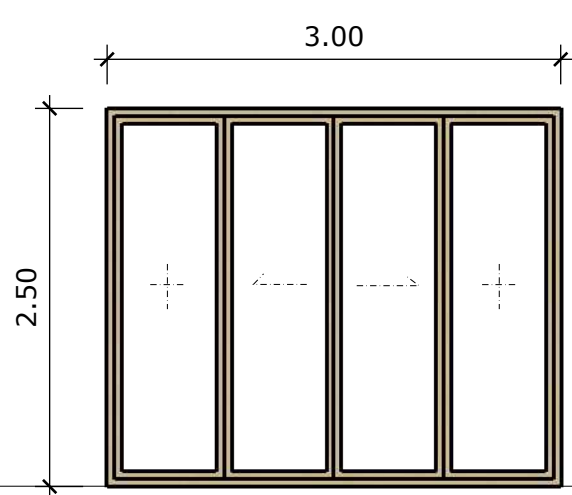
ประตู ①
