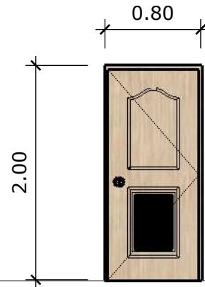
ประตู ②
