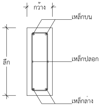
Drawing Title :: รูปตัด A-A scale: No Scale
