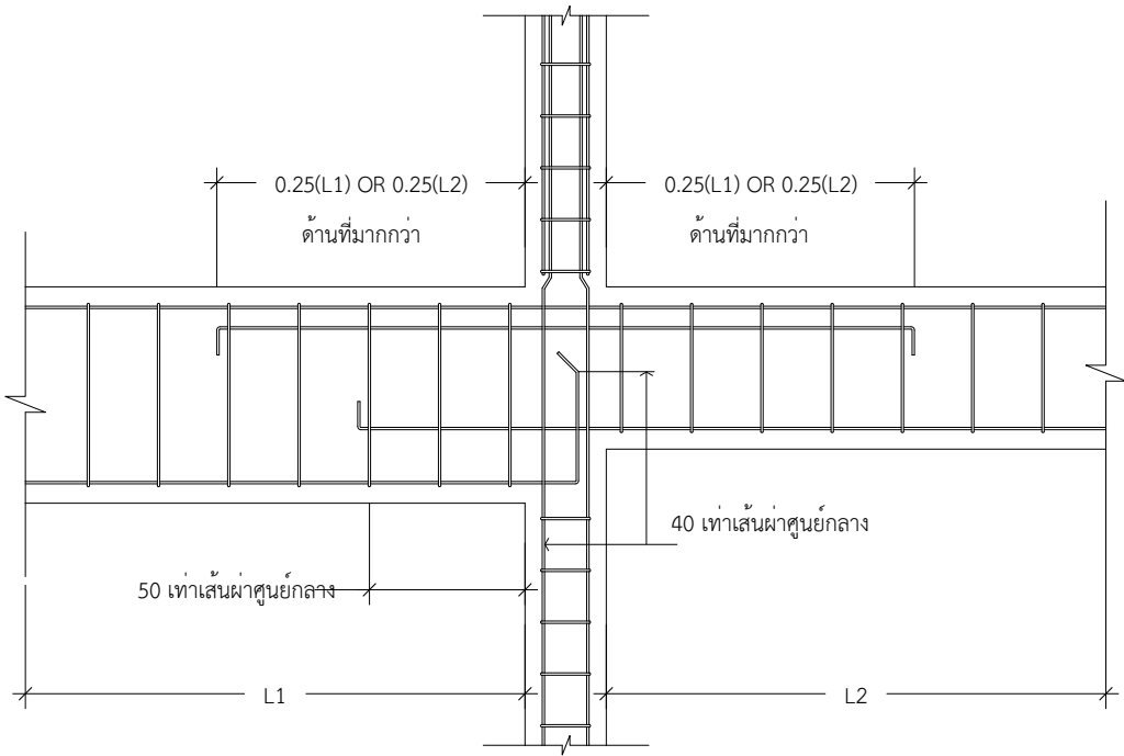
Drawing Title :: มาตรฐานการเปลี่ยนขนาดคาน scale: No Scale
