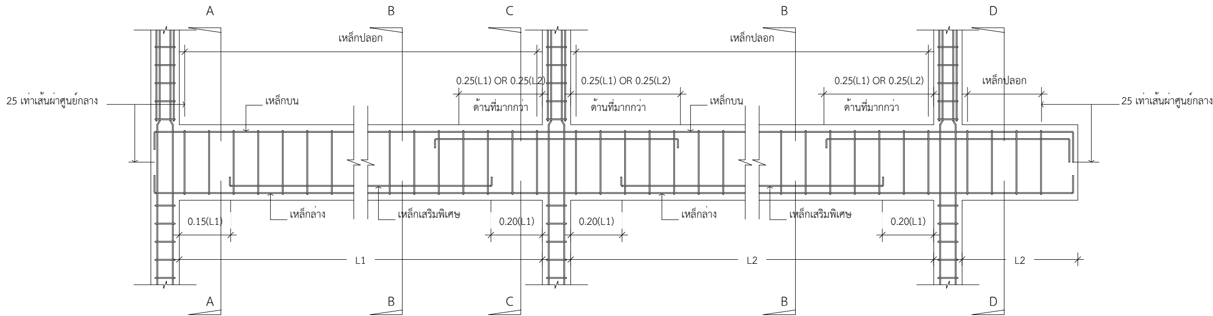
Drawing Title :: มาตรฐานแบบการเปลี่ยนเหล็กเสริมคาน scale: No Scale
