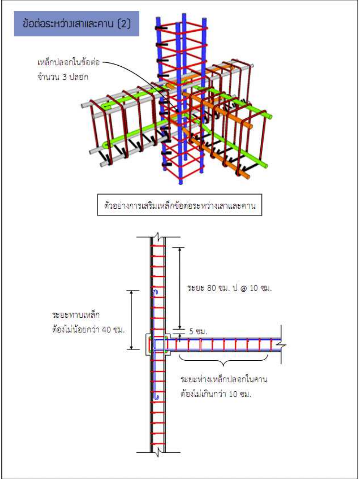
รูปที่ 18 ตัวอย่างรายละเอียดการเสริมเหล็กบริเวณข้อต่อระหว่างเสาและคาน
